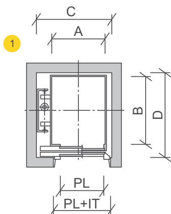
Medidas da cabine e caixa com entrada de um lado
