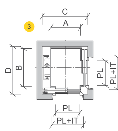
Medidas da cabine e caixa com duas entradas adjacentes
